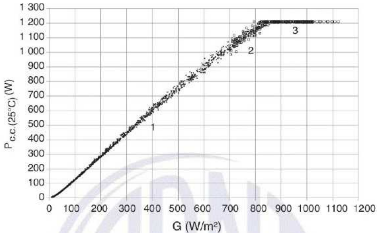
Figura D.1 – Exemplo de curva P_{c.c.}(25^{\circ}C) \times G_C de um arranjo fotovoltaico de 1,5 kWp
