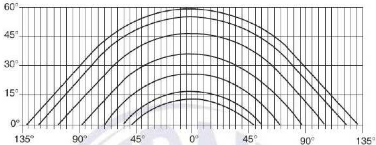
Figura 1 – Diagrama de caminho do sol
