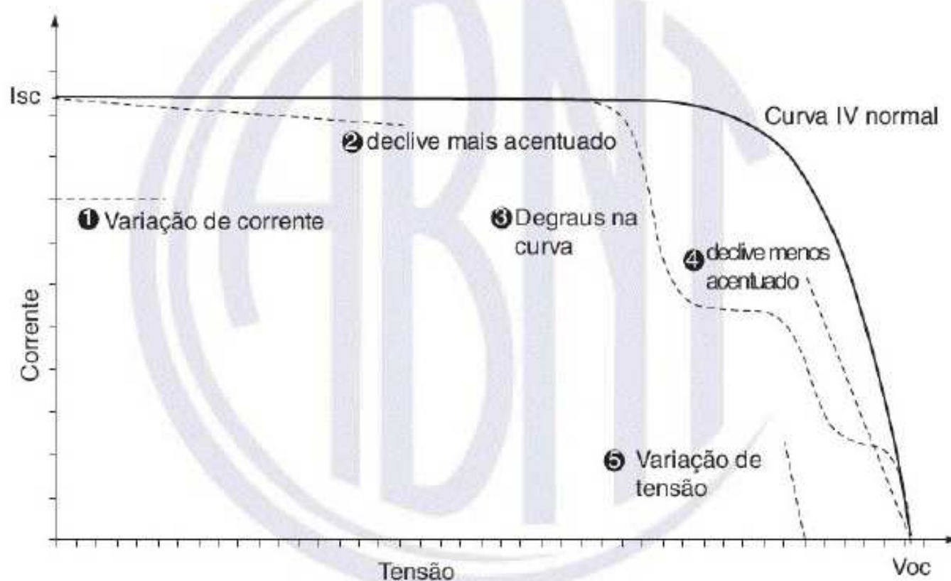
Figura C.1 – Variações na forma da curva IV
