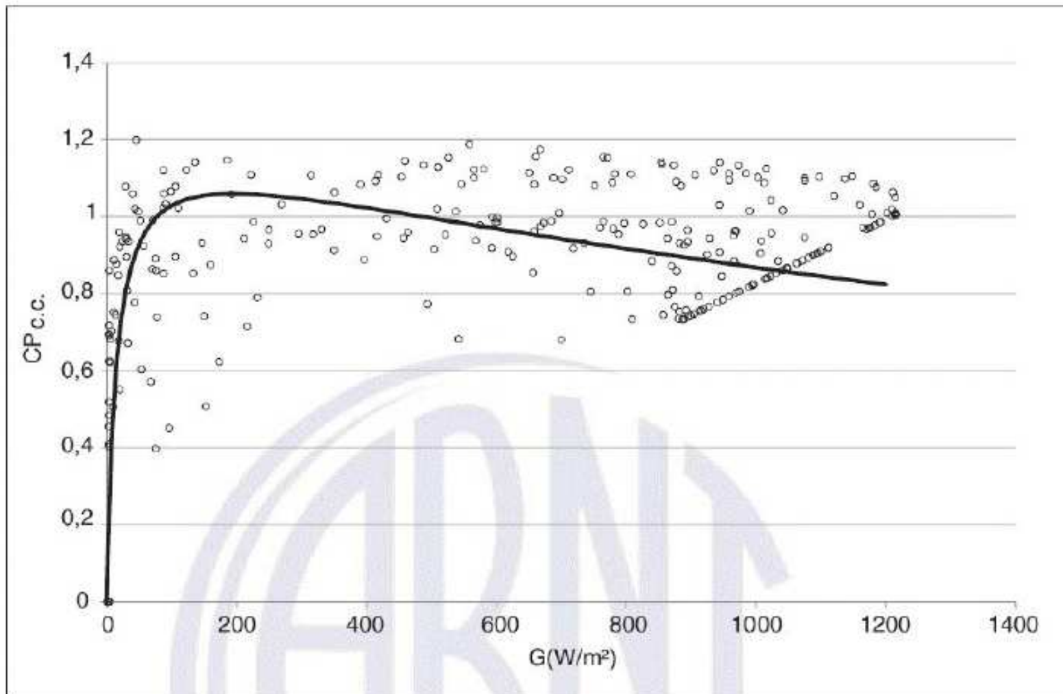
Figura F.2 – Curva do comportamento médio da nuvem de pontos de CP_{c.c.} .
